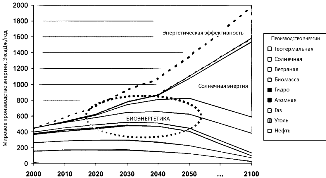
Рисунок 1. Мировые тенденции производства энергоносителей
