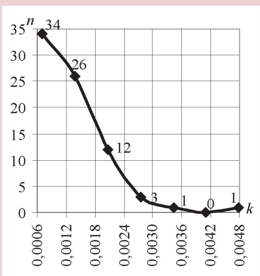
Рисунок 5. Распределение тангенса угла наклона ( k ) линейных функций, построенных для субъектов РФ
