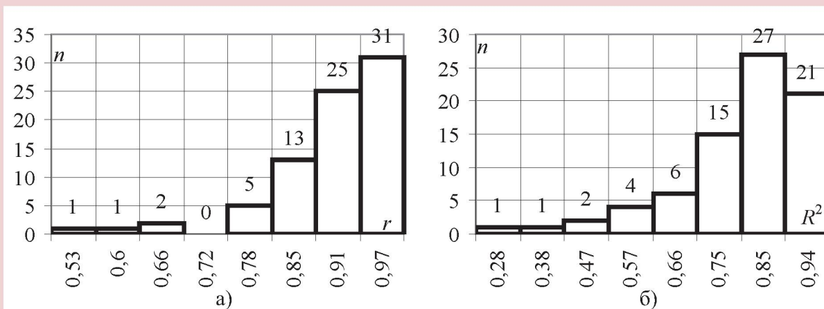
Рисунок 3. Распределение значений показателей для оценки достоверности: а) коэффициент корреляции (Пирсона, r ); б) среднеквадратичное отклонение линейных функций ( R^2 )
