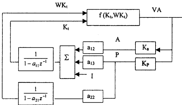
Рис. 3. Модель воспроизводственного процесса на уровне отрасли
