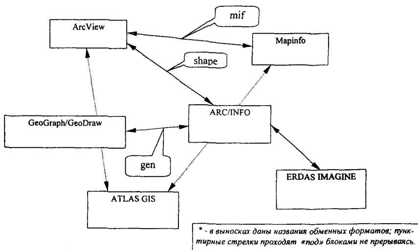
Рис. 2.7. Схема конвертации данных при обмене между наиболее популярными ГИС
